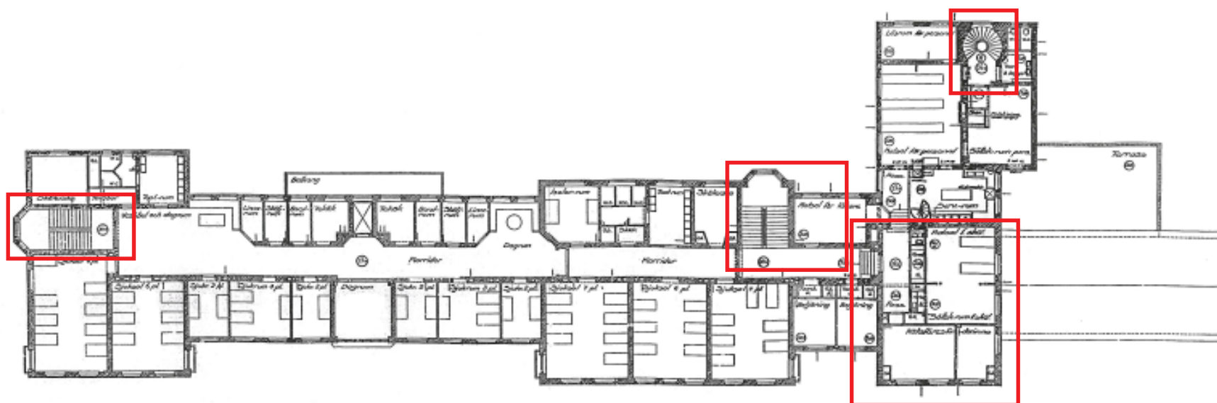
Ovan: Våning 2 tr 1936. På planen är värdefulla enheter markerade. Nedan: Våning 3 tr 1936. På planen är värdefulla enheter markerade.
