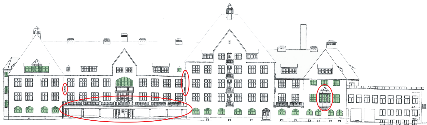
Södra fasaden med original- samt äldre fönster grönmarkerade och värdefulla detaljer rödmarkerade.
