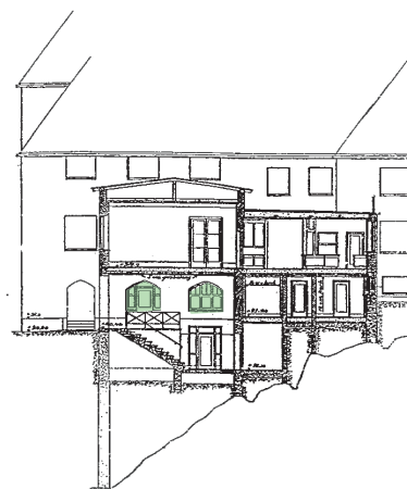
Norra fasaden med original- samt äldre fönster grönmarkerade.
